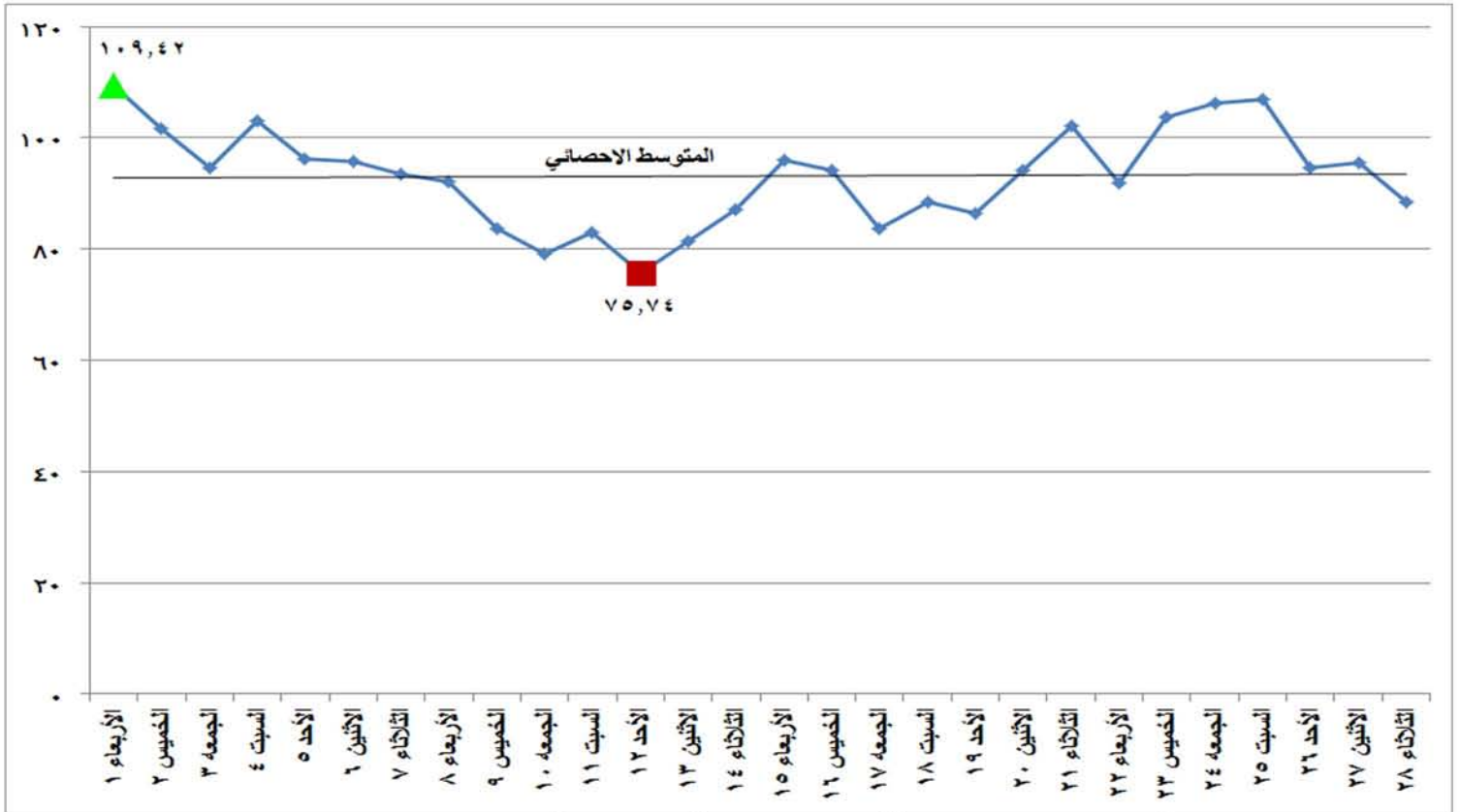
شكل (١٩) الطاقة الكهربائية المنتجة من المازوت خلال شهر فبراير ٢٠١٧
