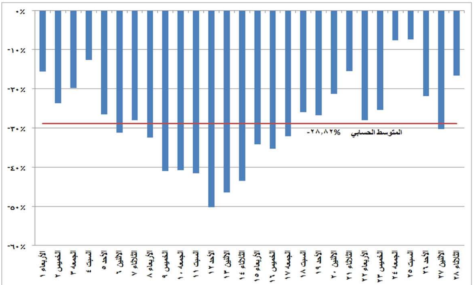
شكل (٢٠) نسب التغير في استخدام المازوت في إنتاج الطاقة الكهربائية خلال شهر فبراير ٢٠١٧ مقارنة بالشهر المماثل من العام السابق
