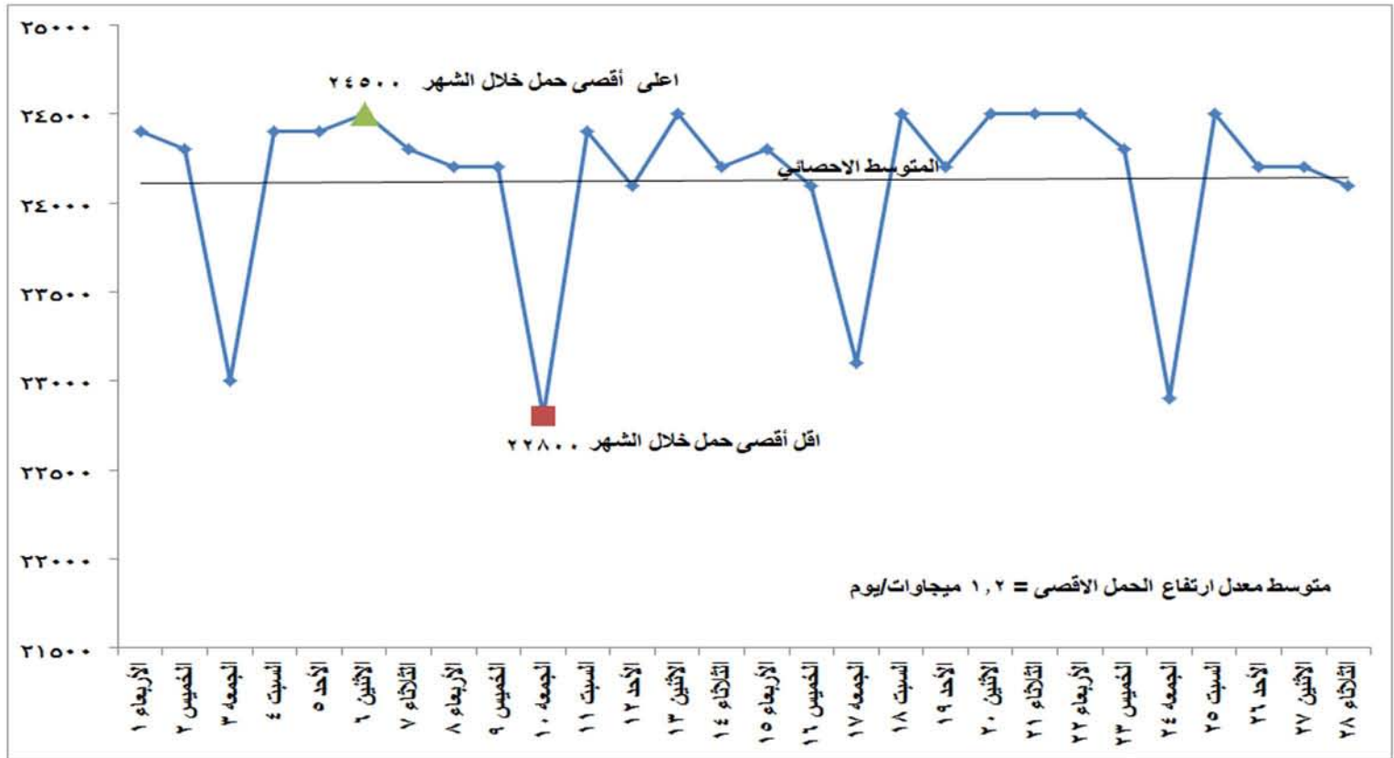
شكل (١) تطور الحمل الاقصى اليومي خلال شهر فبراير ٢٠١٧
