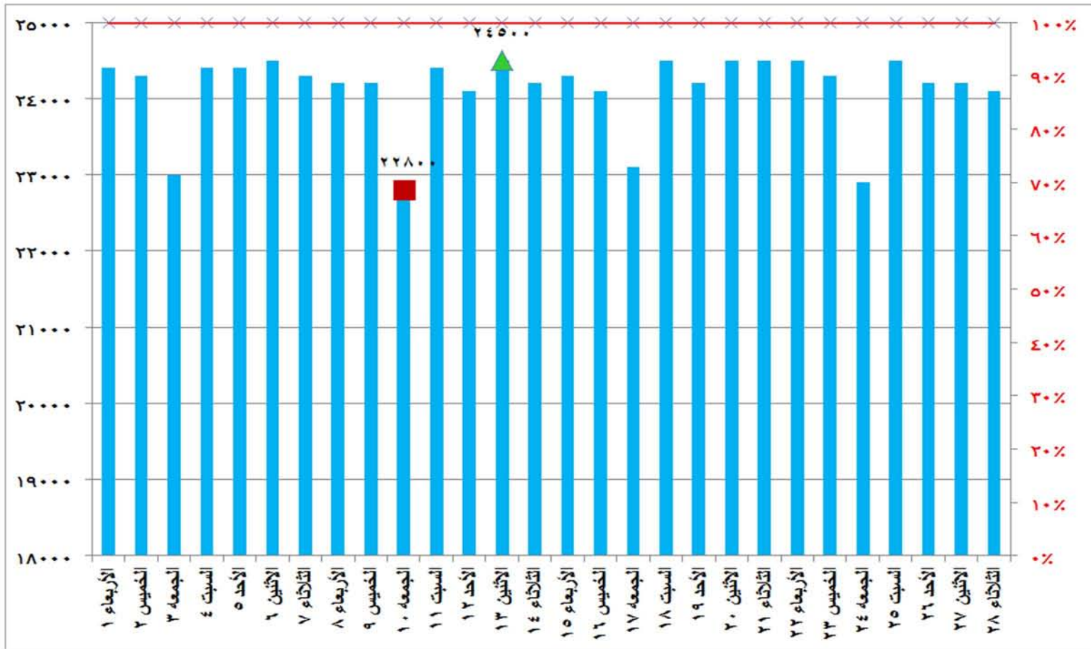
شكل (٥) قدرات الانتاج المتاحة ونسبتها للحمل الأقصى خلال شهر فبراير ٢٠١٧
