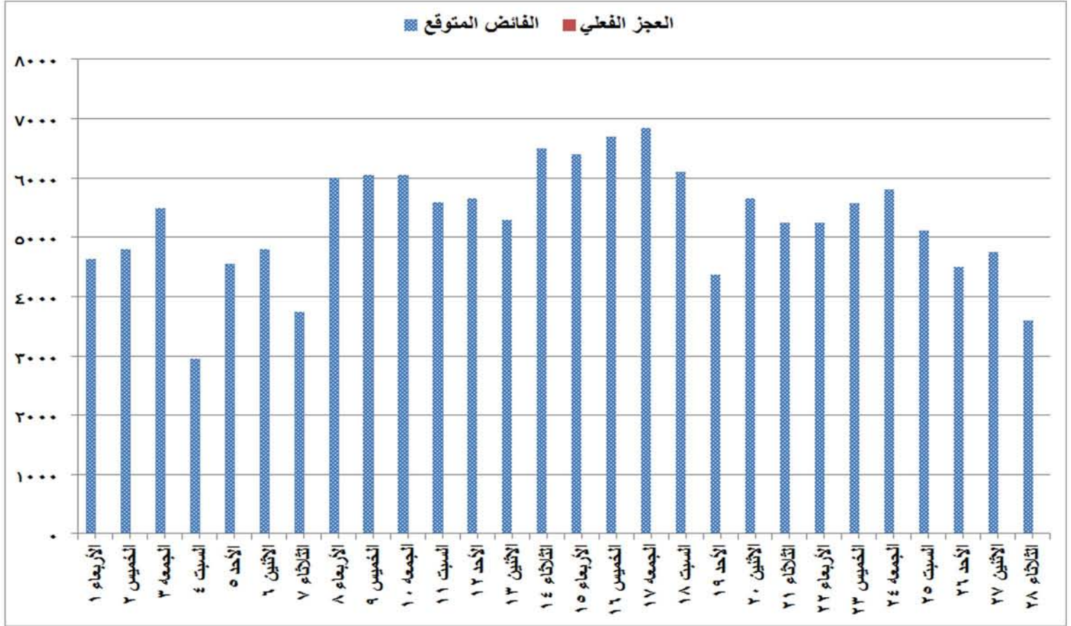
شكل (٧) الفاوض والعجز المتوقع للقدرات خلال شهر فبراير ٢٠١٧
