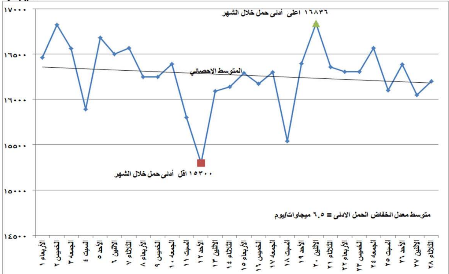
شكل (٢) تطور الحمل الادنى اليومي خلال شهر فبراير ٢٠١٧
