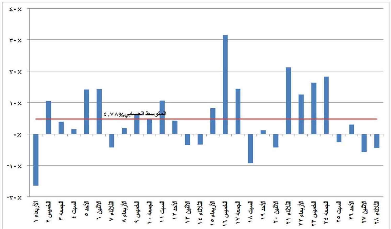
شكل (٢٢) نسب التغير في استخدام المصادر غير الحرارية في إنتاج الطاقة الكهربائية خلال شهر فبراير ٢٠١٧ مقارنة بالشهر المماثل من العام السابق
