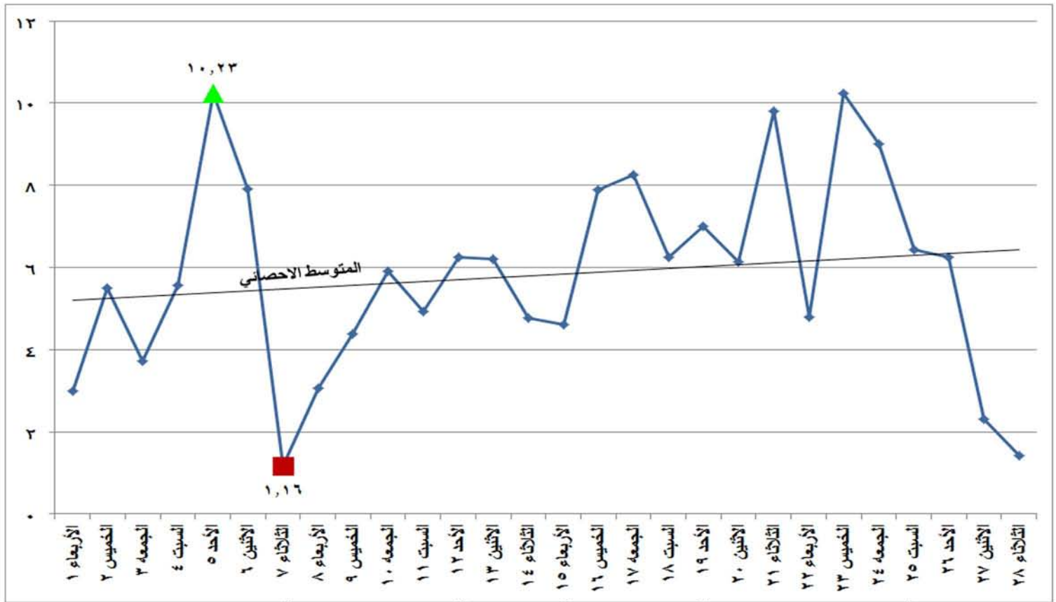
شكل (٢٥) الطاقة الكهربائية المنتجة من الرياح والشمس خلال شهر فبراير ٢٠١٧
