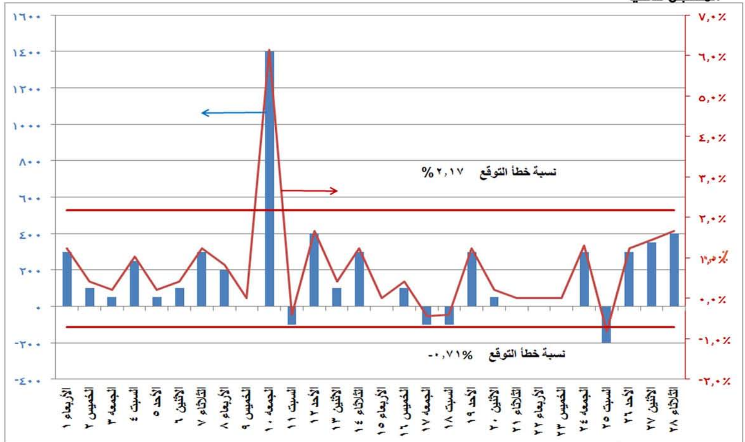
شكل (١٠) الفرق بين الحمل الأقصى المتوقع والمسجل فعلياً ونسبة الفرق إلى الحمل المسجل فعلياً خلال شهر فبراير ٢٠١٧
