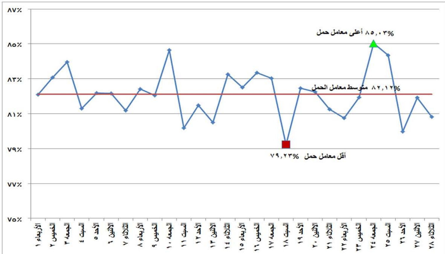
شكل (١٢) إجمالي معامل الحمل لوحدات الانتاج خلال شهر فبراير ٢٠١٧
