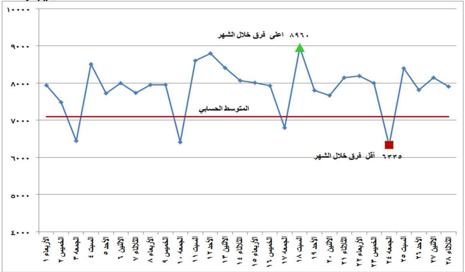
شكل (٣) الفرق بين أقصى وأدنى حمل خلال شهر فبراير ٢٠١٧
