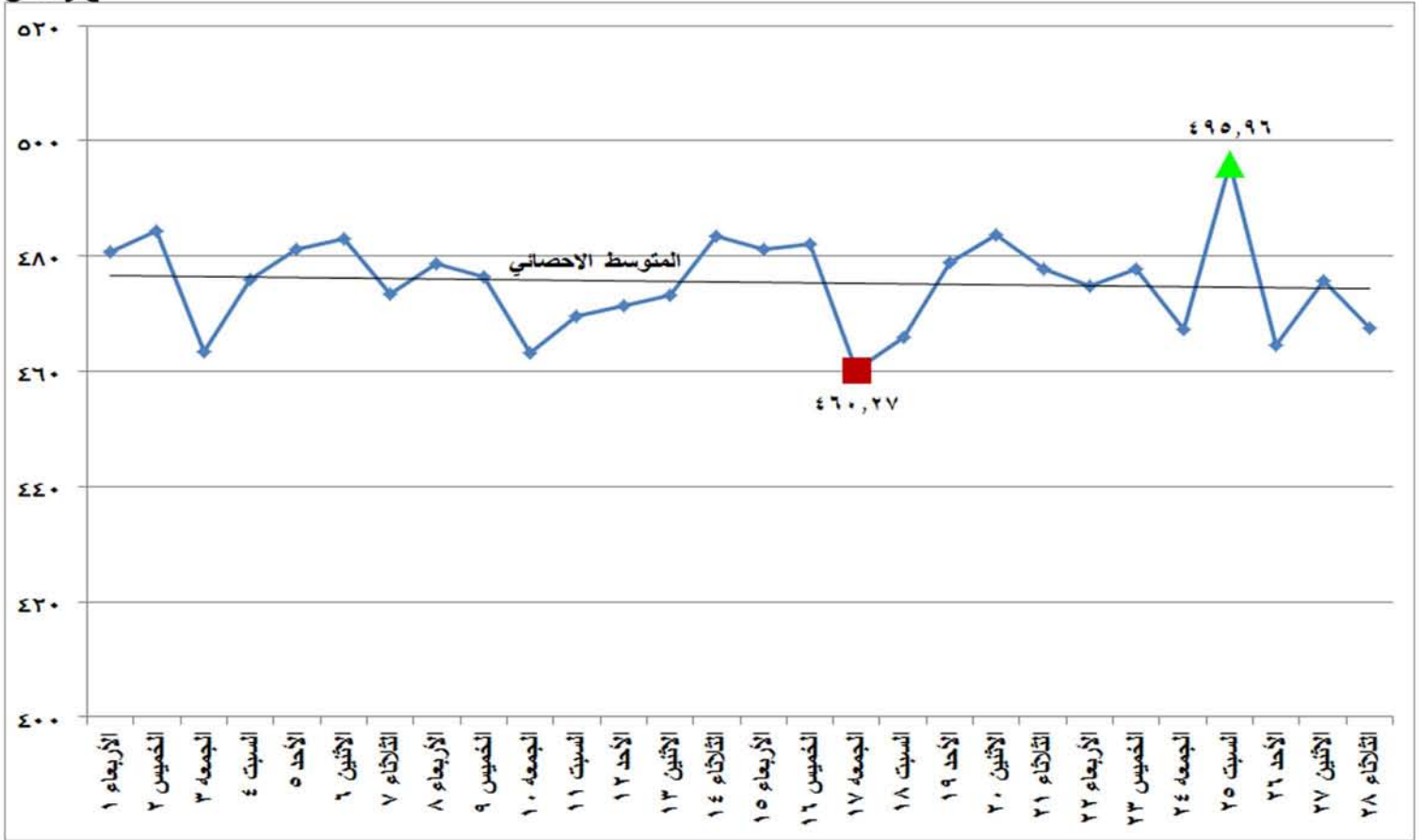
شكل (١٥) إجمالي الطاقة الكهربائية المنتجة من كل المصادر الأولية خلال شهر فبراير ٢٠١٧
