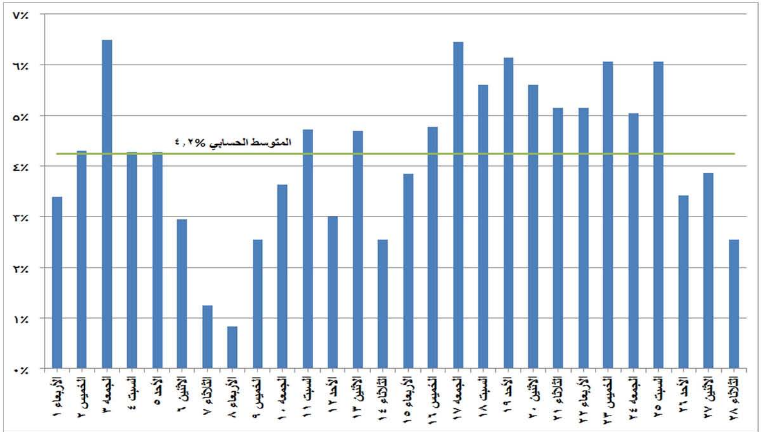
شكل (٩) النسب المئوية للتغير في الحمل الأقصى خلال شهر فبراير ٢٠١٧ مقارنة باليوم المماثل من العام الماضي
